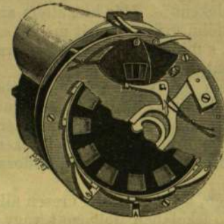
A gépezet részletei.
