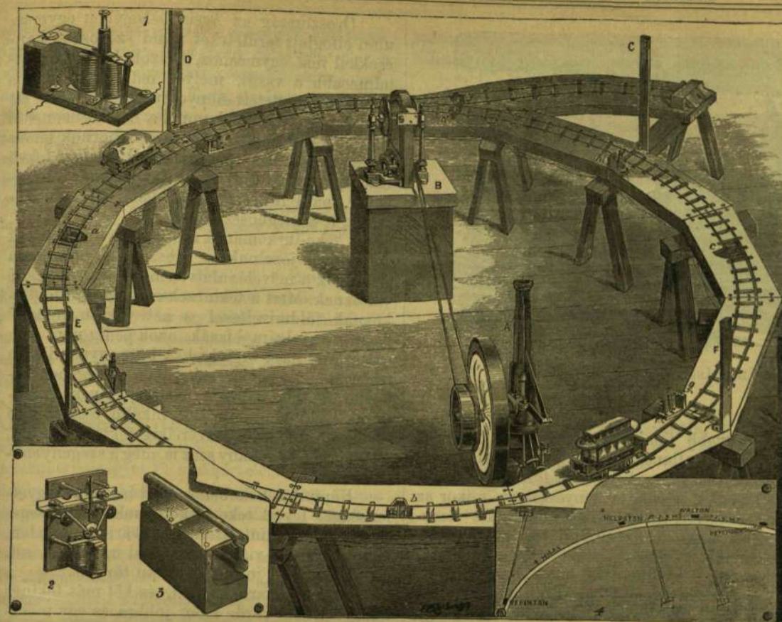
A gőzgépe mint hajtóerő. — B villamosság-gerjesztő gép. C D E F villamos indikátorok. — a b c d érintkezést közvetítő, mindegyik szelvény végén. — e f g h elektromágnesek, mindegyik szelvény számára. — 1. Ugyanezen elektromágnes nagybójtva. — 2. Érintkezést közvetítő. — 3. Ugyanez a sínekre alkalmazva. — 4. Mappa, mely megmutatja, hol halad a vonat.
